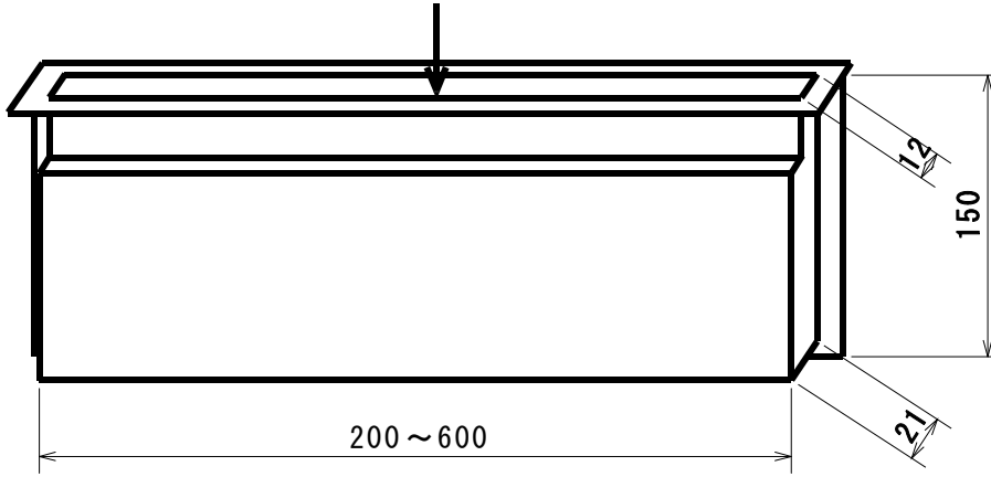
タンク部
